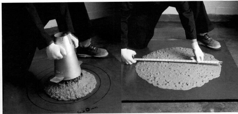
Figura 1 – Ensaio de espalhamento.
